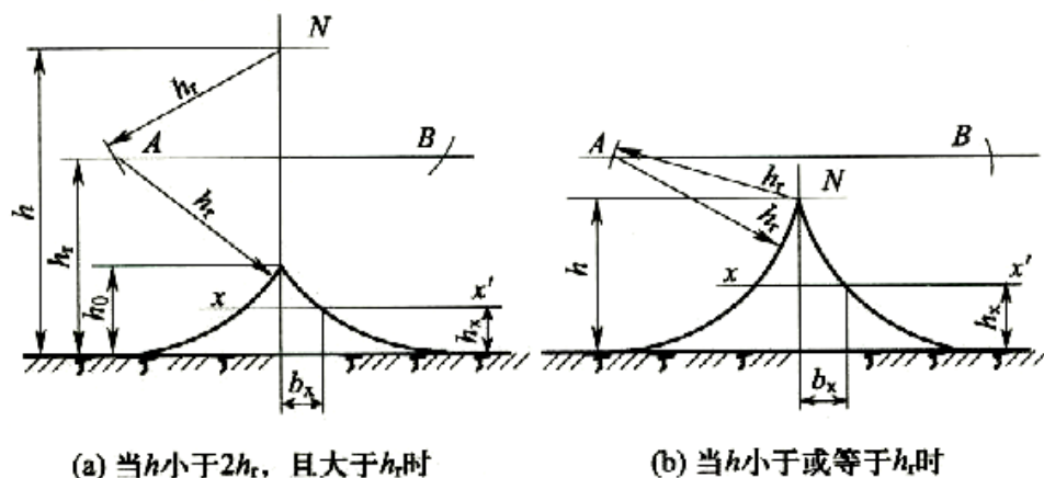
图 D.0.5 单根架空接闪线的保护范围
