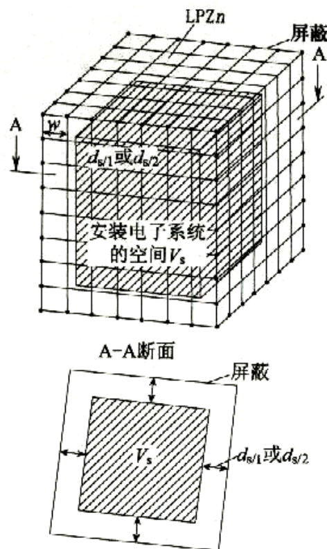
图 6.3.2-2 在 LPZn 区内供安放电气和电子系统的空间
