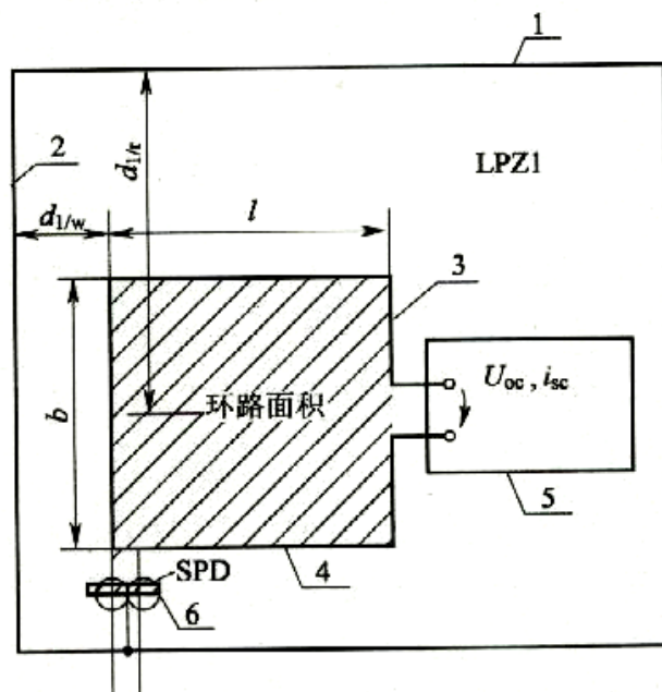
图 G.0.1 环路中的感应电压和电流
